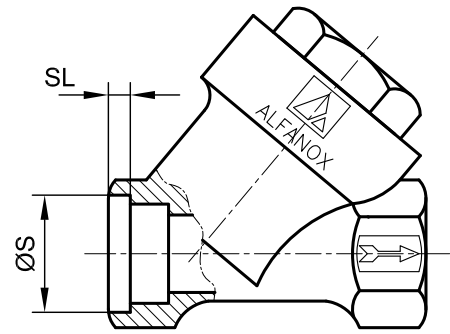
KAYNAK SOKETLİ
