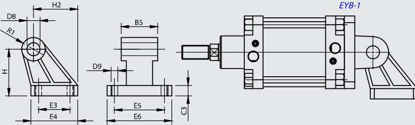
YB Yer Bağlantı
