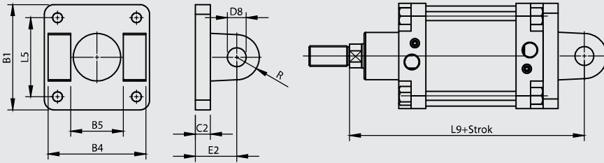
YB Yer Bağlantı
