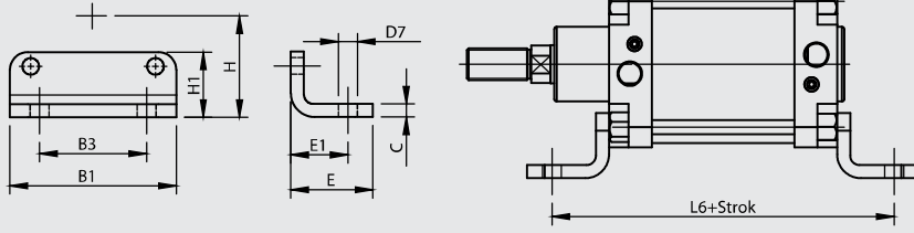
AB Ayak Bağlantı
