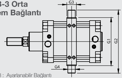
OEB-3 : Ayarlanabilir Bağlantı
